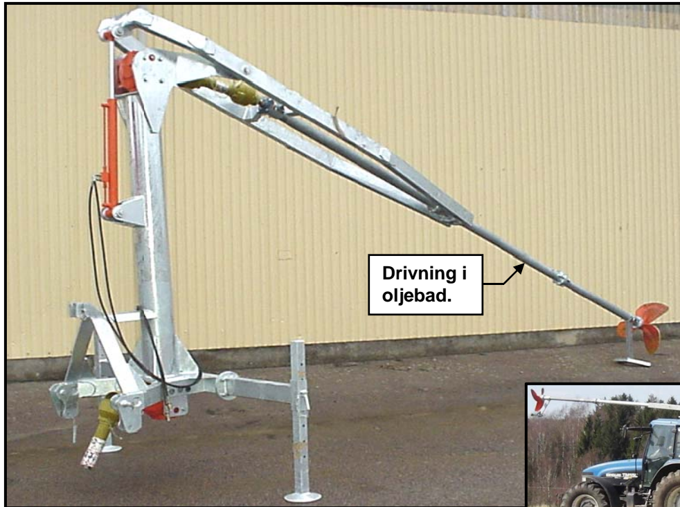
Modell ALPI för 2 - 4,5 m höga brunnar
